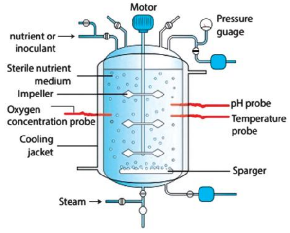
Bioreactor
