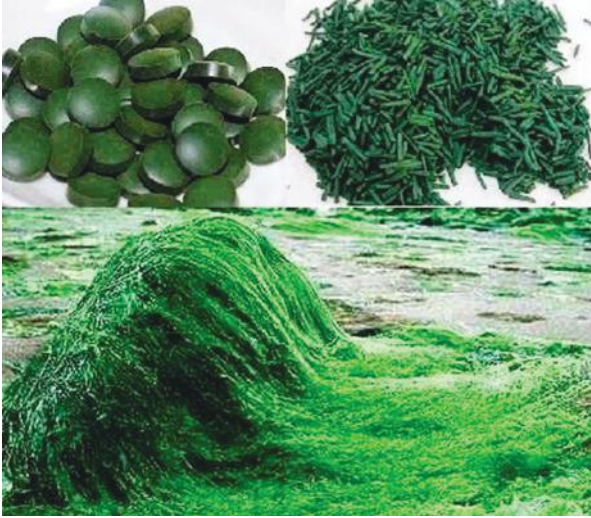
Spirulina
